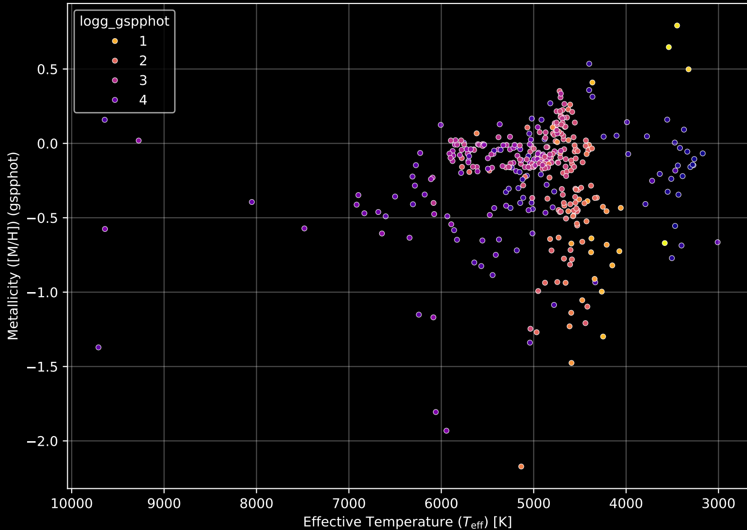
APOGEE DR17 Field: [K2_C7_009-18] Stellar Population Parameters (n= 366)
